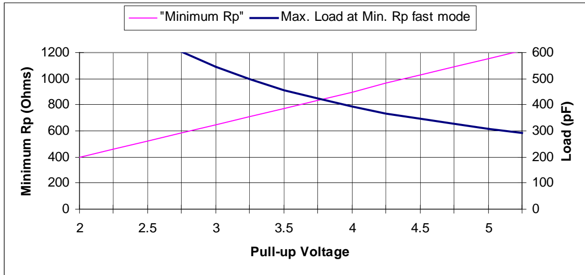
图 12. 高速 I 2 C 模式下的上拉电阻选择
