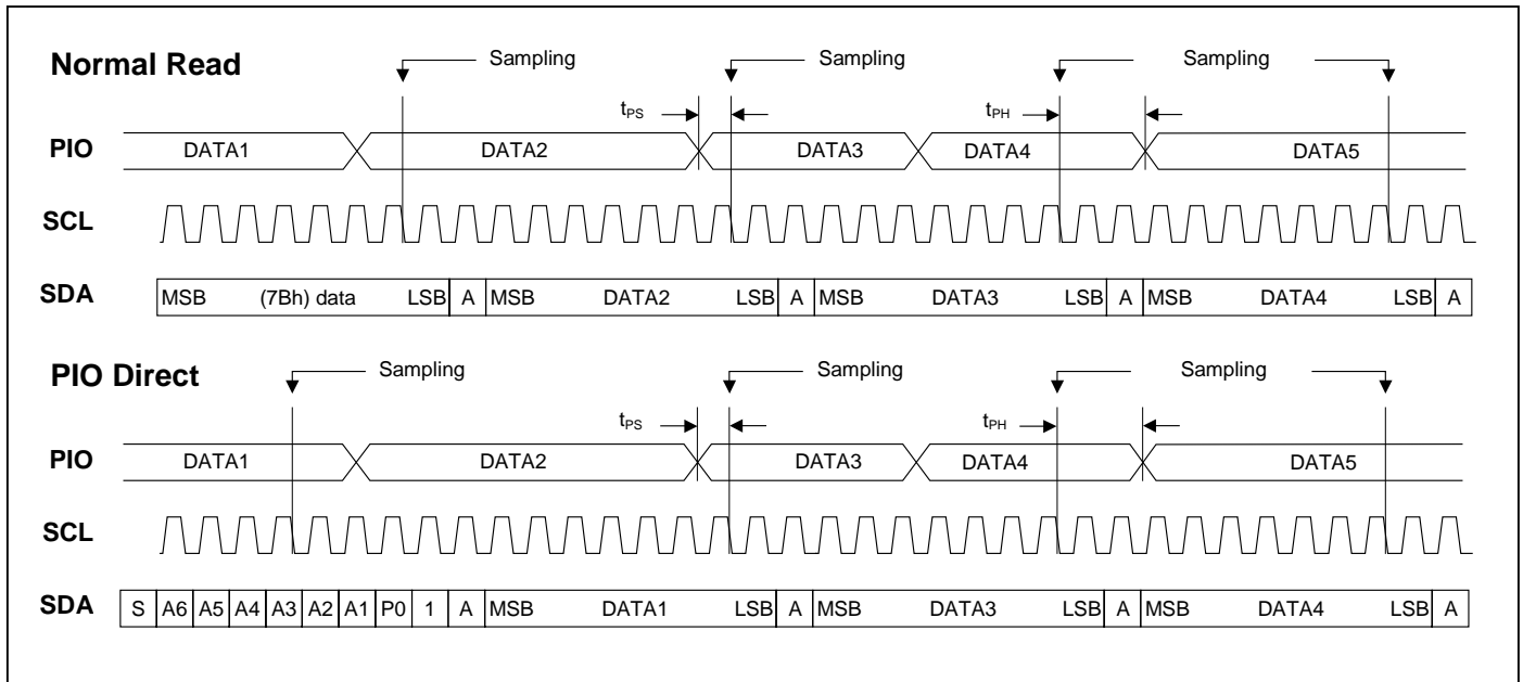
图 10. PIO 读访问时序
