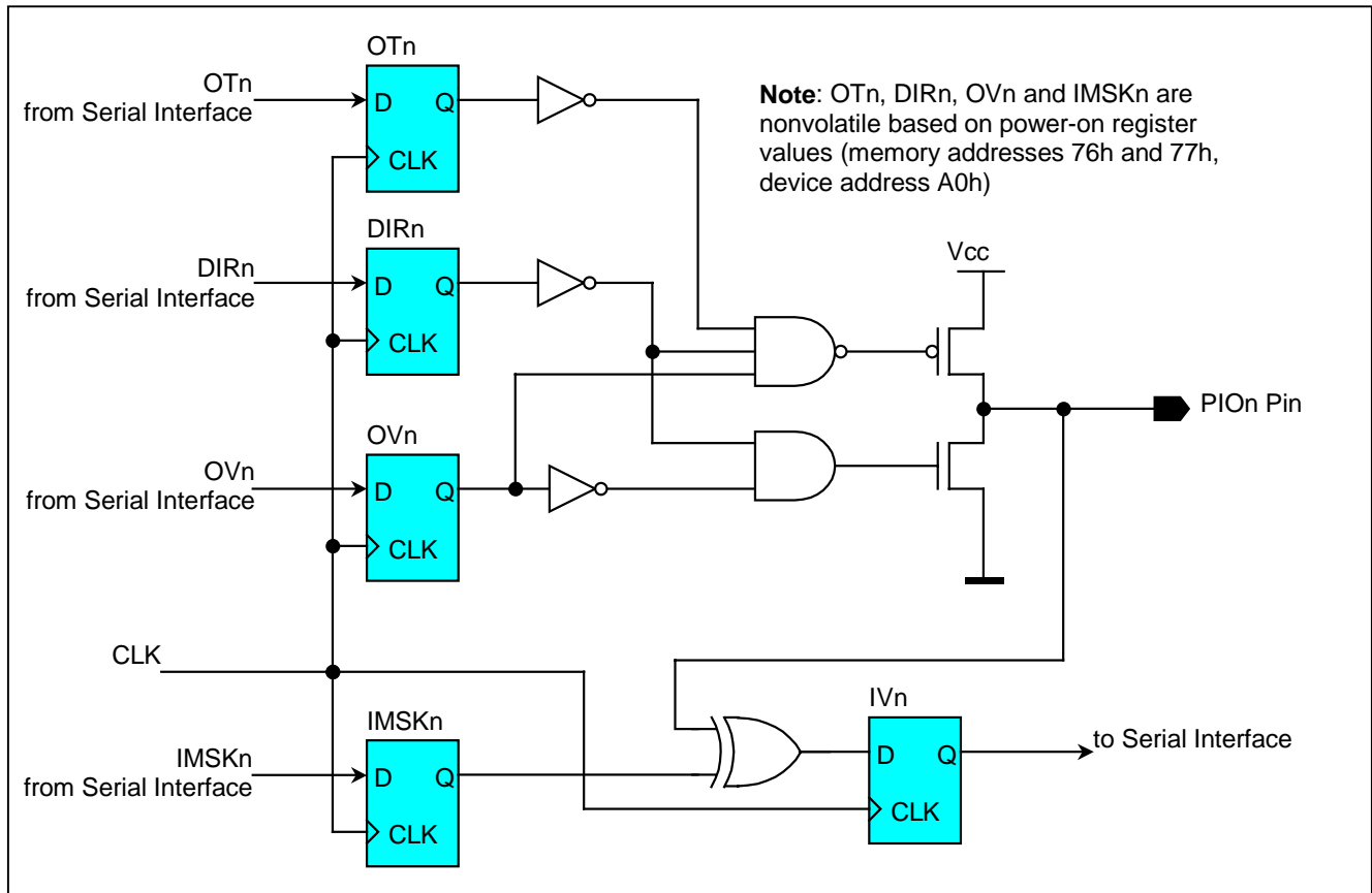
图 3. PIO 简化原理图
