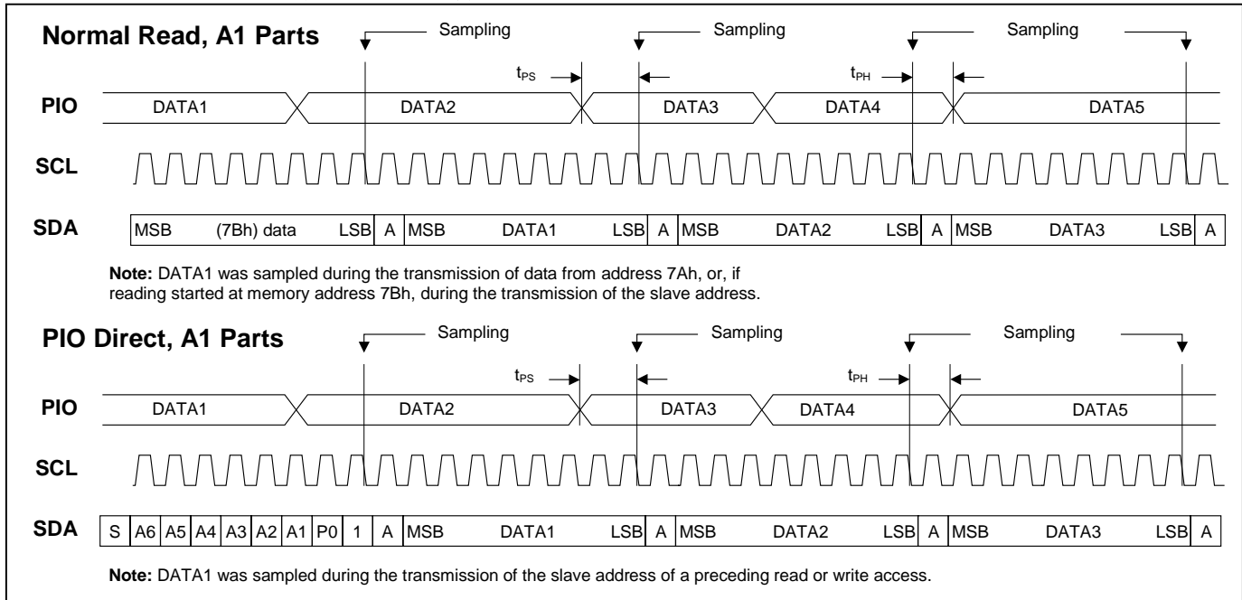
图 10A. PIO 读访问时序, A1 版器件
