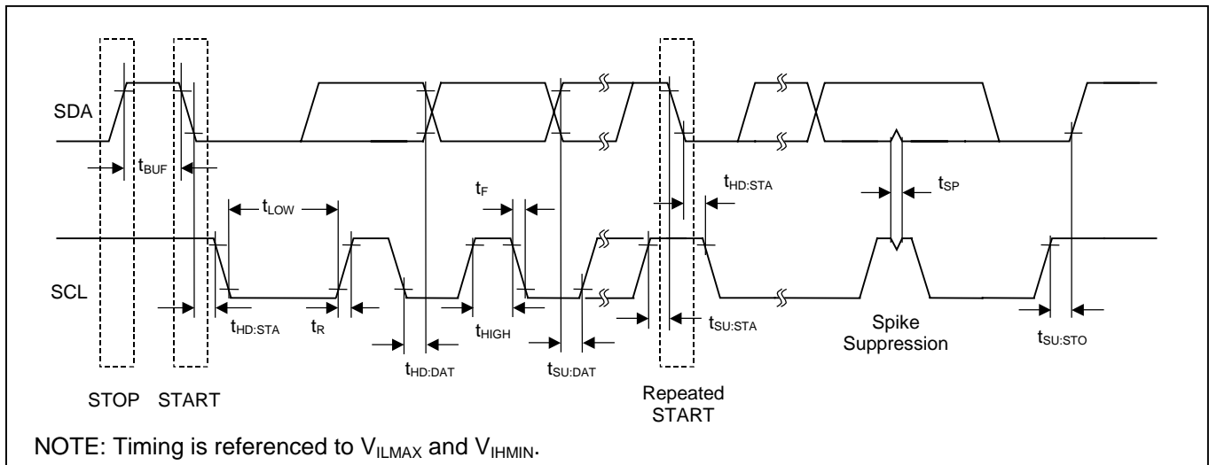
图 6. I 2 C/SMBus时序图
