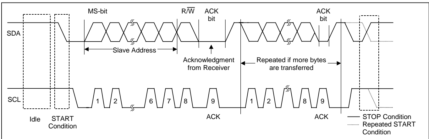
图 5. I 2 C/SMBus 协议
