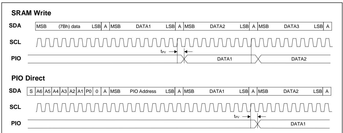
图 8. PIO 写访问时序
