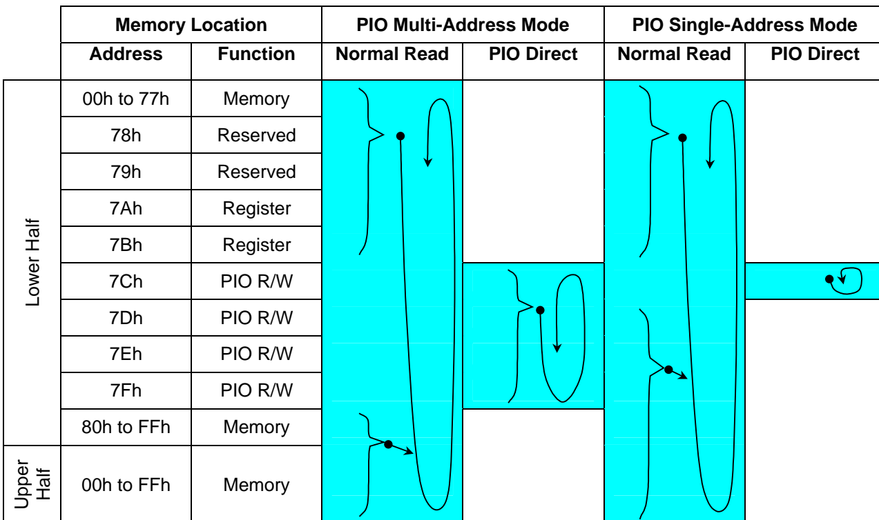
图 9. 存储器和 PIO 读序列
